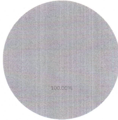
Curva ABC
